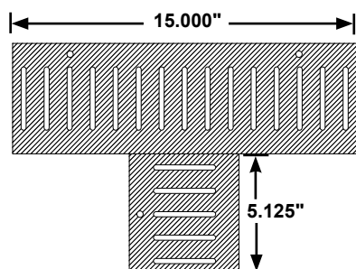
QP-6257 Universal Tee
